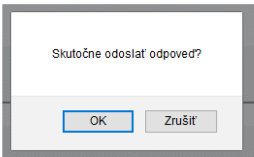
Obrázok 28 - Potvrdzujúce okno
